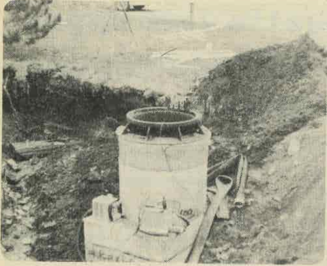
Les travaux de la pose des tuyaux d'égoûts dans le rang double sont commencés. Ces travaux sont sous la direction du Surintendant de la Voirie de la Municipalité, M. René Collins. Il voit à l'engagement des hommes et de la machinerie nécessaire. Les raccords se feront au printemps prochain.
