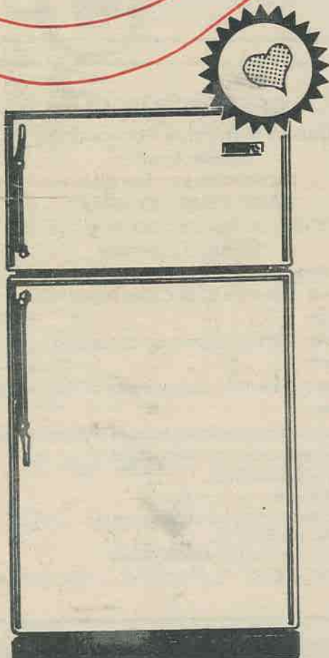
RFS-15 Réfrigérateur Sans-Givre Satellite. Moteur-compresseur garanti 10 ans. Capacité totale 15 pi. cu. Réfrigérateur 11 pi. cu. Congélateur 4 pi. cu. 2 clayettes réglables 10 positions. Compartiment à beurre. 2 oeufriers et 2 bacs à glaçons. 8 balconnets de portes. Roulettes arrières. Nouvel isolant réduit la consommation d'électricité.
